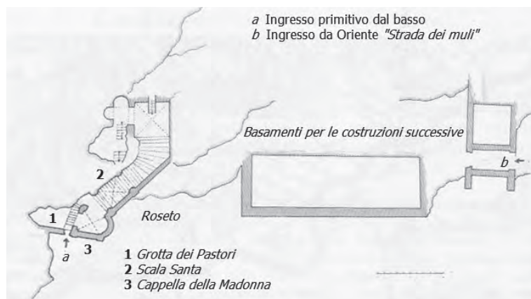
Fig. 5 - Planimetria con evidenziato il primitivo ingresso al Sacro Speco, che avveniva dal basso, le due grotte rappresentative, la Scala Santa e gli imponenti basamenti per le successive fasi costruttive.
