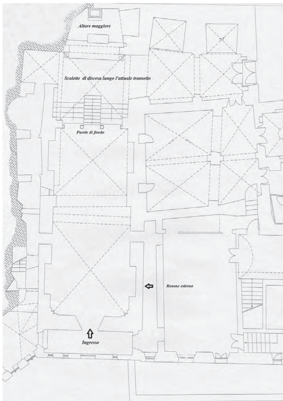
Fig. 15 - Planimetria della chiesa superiore del Sacro Speco con le superfici laterali.
