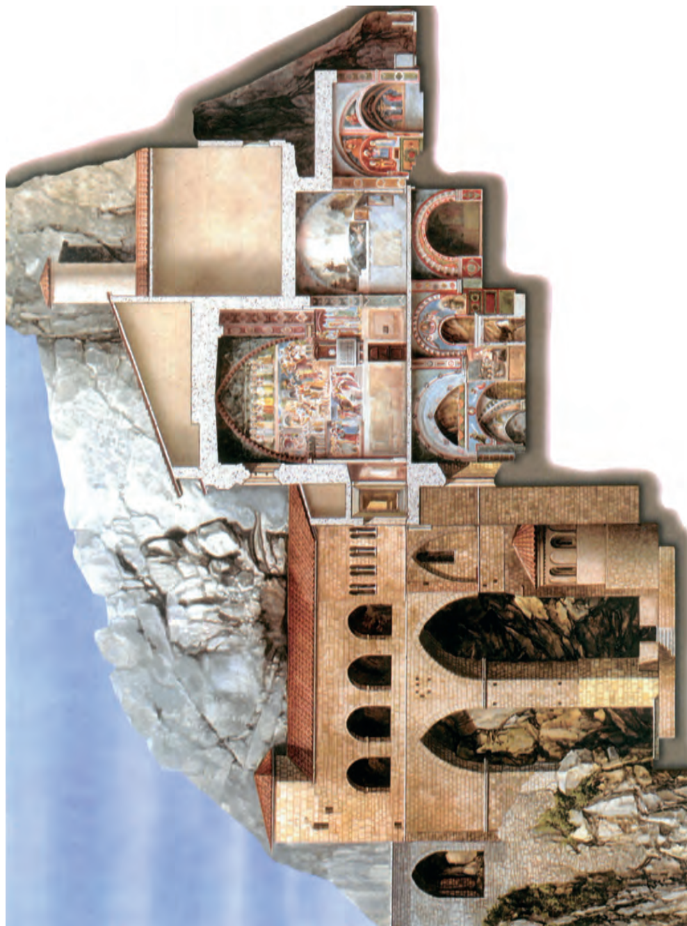
Fig. 4 - Sezione della chiesa inferiore e superiore con vista della parte Ovest realizzata per accedere, dall'alto, a tutto il Santuario.
