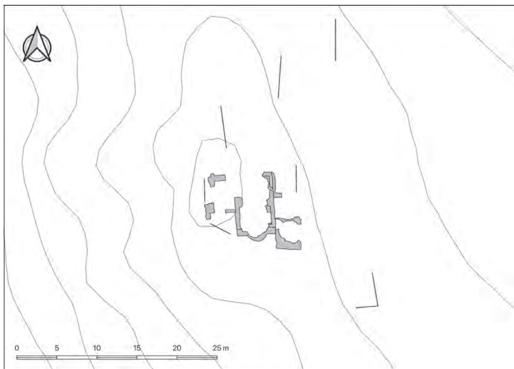
Fig. 7 - Rilievo delle strutture individuate sull'anticima del Monte Gennaro. In nero i resti di allineamenti murari visibili sul terreno ma non conservati in elevato (elaborazione grafica: Matteo Rossi).
