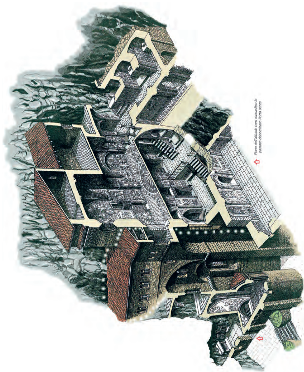
Fig. 8 - Spaccato dal quale si riscontra (dalla freccia in rosso) l'ingresso originario al Monastero. A tratteggio (con punti in bianco) la realizzazione del nuovo ingresso dall'alto che ha consentito di accedere frontalmente alla chiesa superiore, eliminando un affresco.
